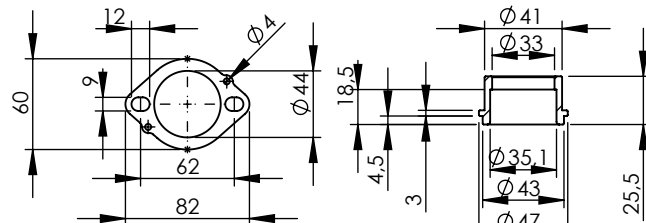
S.s Flange 112A cod.204569 Sp.5mm
